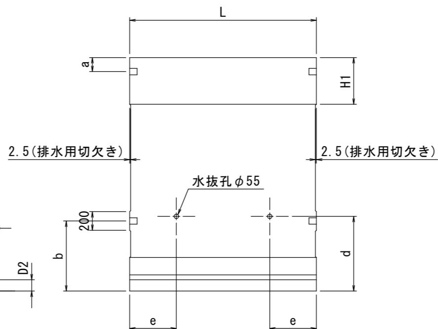
背面図
