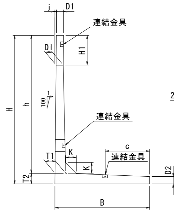
側面図
